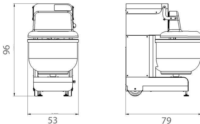
Dimensions maximum de la RS48 en cm.
