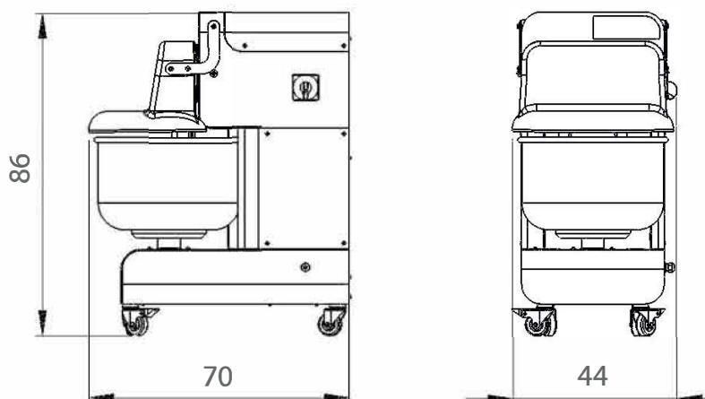
Dimensions maximum de la RS12 en cm.
